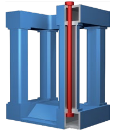
Das Walzengestell: Mehrteilig ausgebildet und durch Zuganker vorgespannt
