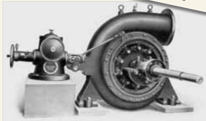
Francis-Spiralturbine mit liegender Welle
